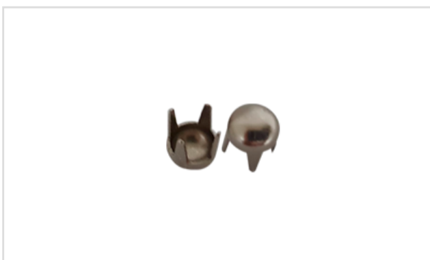
ANTRAG: Cravo 4,5 Redondo BESCHREIBUNG: Carnation 4.5 Rund MATERIAL: Eisen oder Messing DIMENSIONEN: 4,5mm (kopf)
