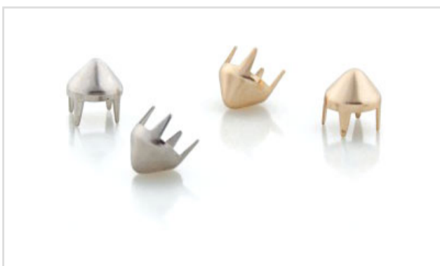
ANTRAG: Cravo 7,0 Ponta (SPIKE) BESCHREIBUNG: Carnation 7.0 Spike Point MATERIAL: Eisen oder Messing DIMENSIONEN: 7mm (kopf)
