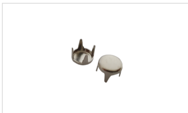
ANTRAG: Cravo 6,0 Chato BESCHREIBUNG: Crab 6.0 Boring MATERIAL: Eisen oder Messing DIMENSIONEN: 6,0mm (kopf)
